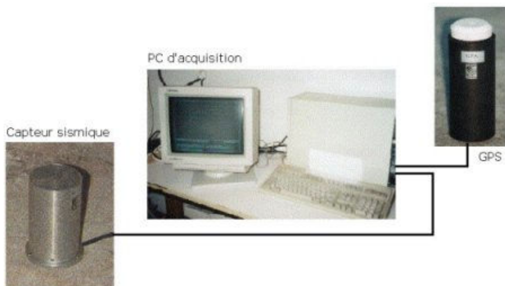
Station sismologique à vocation éducative
